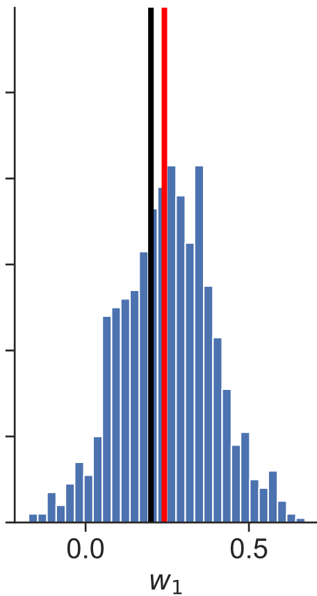
Posterior distributions Dataset 17
