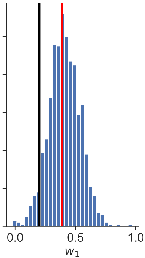
Posterior distributions Dataset 37
