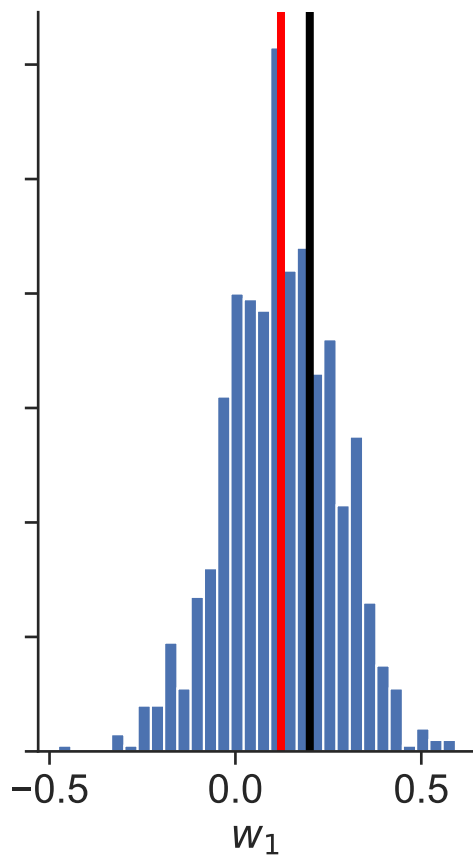
Posterior distributions Dataset 32
