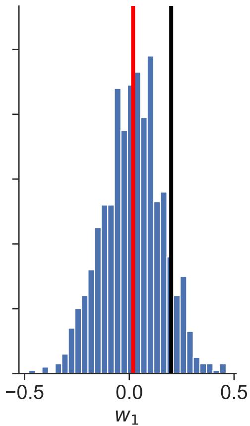
Posterior distributions Dataset 26
